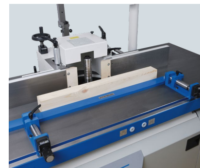
Gegenanschlag
