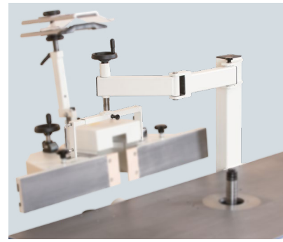
Abschwenkvorrichtung für Fränschlag
