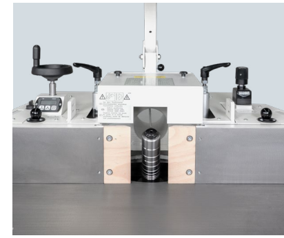
Fränschlag Typ 2620 mit Gussanschlagbacken, AIR-LOCK
